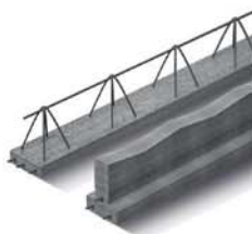
BELKI STROPOWE
